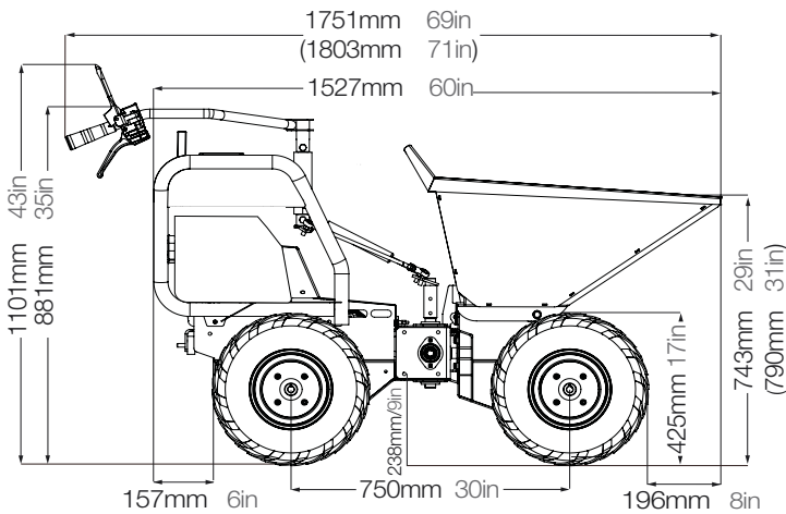
Afmetingen B300 BENDie (B450 BENDie)
